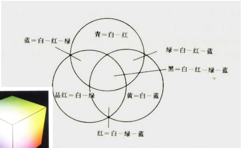
CMY
