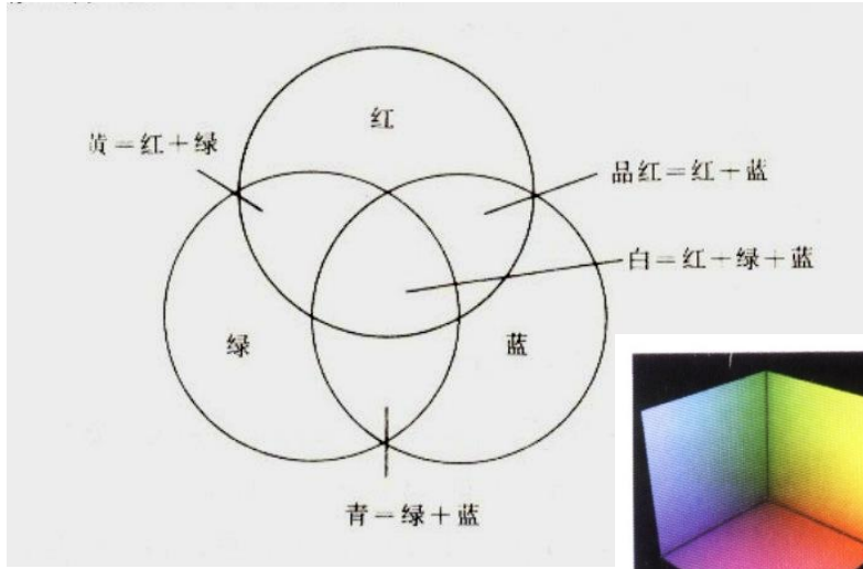
RGB
