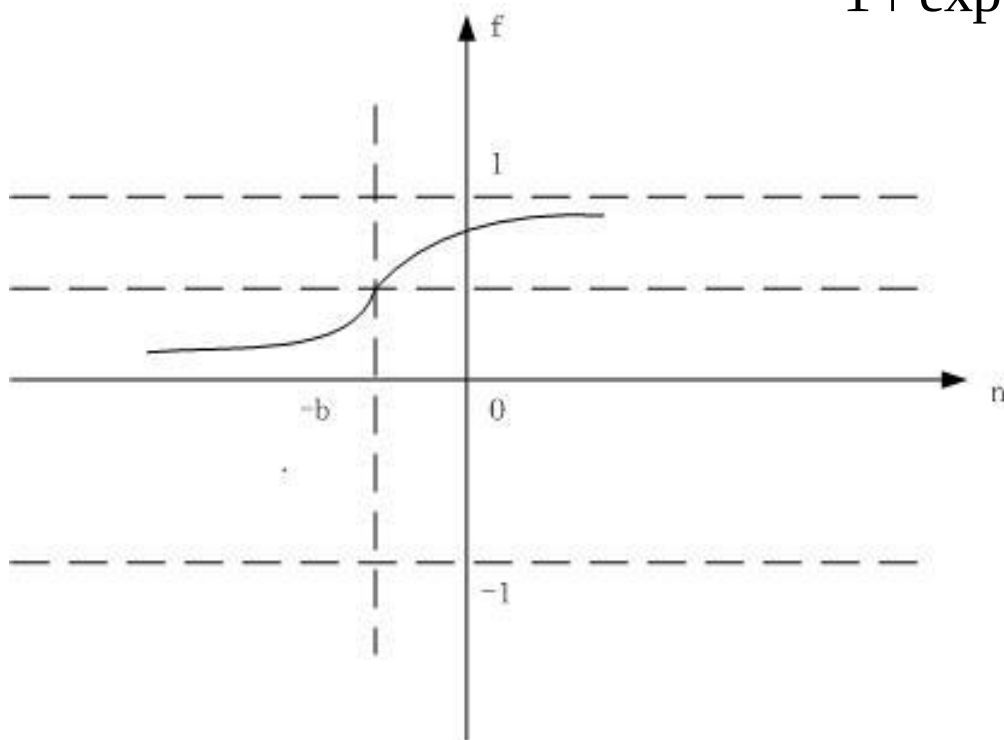
带有偏差的对数S型激活函数
